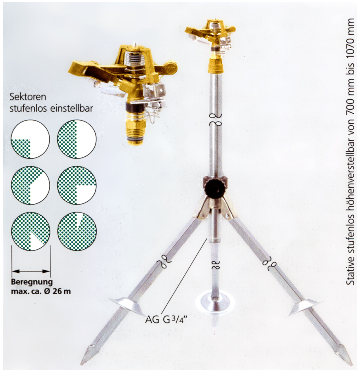
Stativregner
